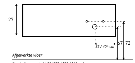
Aan- /afvoer PITCH Rechts 100 / 120 / 140 / 160 (designsifon laag model)
