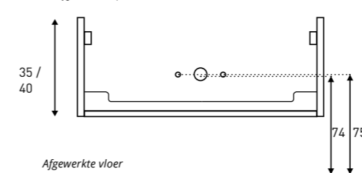
Aan- /afvoer FAKTOR/ASPEKT Midden 60 / 80 / 100 / 120 / 140 (bijgeleverde platte sifon)
