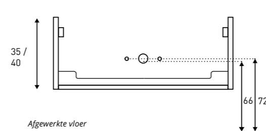
Aan- /afvoer PITCH Midden 60 / 70 / 80 / 90 / 100 / 120
