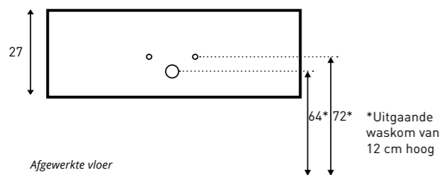
Aan- /afvoer TOPDECK 60 / 70 / 90 / 100 / 120 / 140
