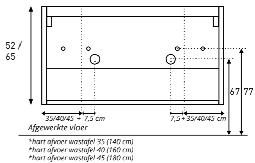
Aan- /afvoer POST Dubbel 140 / 160 / 180
