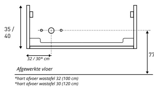
Aan- /afvoer POST Links 100 / 120 (bijgeleverde platte sifon)
