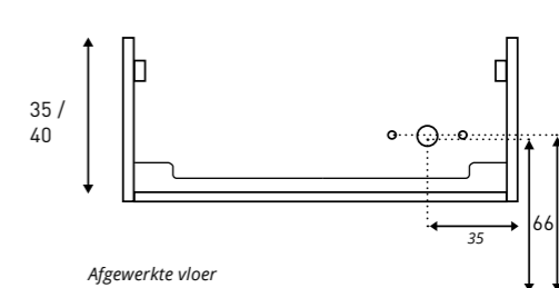
Aan- /afvoer PITCH Rechts 100 / 120
