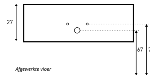
Aan- /afvoer PITCH Enkel 60 / 80 / 100 / 120 (designsifon laag model)
