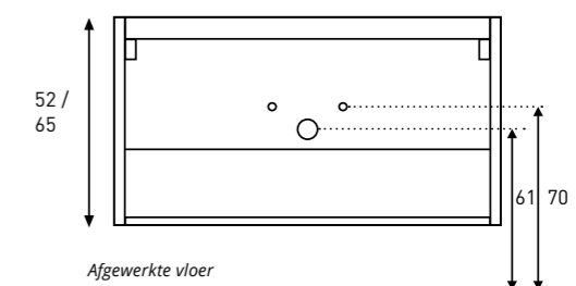
Aan- /afvoer UNITED 60 / 70 / 80 / 90 / 100 / 120 / 140
