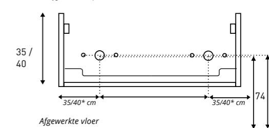
Aan- /afvoer FAKTOR/ASPEKT Dubbel 140 / 160 (bijgeleverde platte sifon)
