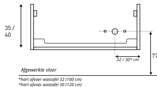
Aan- /afvoer POST Rechts 100 / 120 (bijgeleverde platte sifon)
