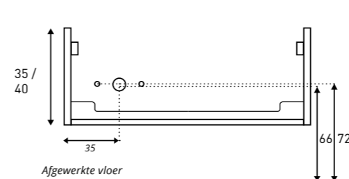
Aan- /afvoer PITCH Links 100 / 120
