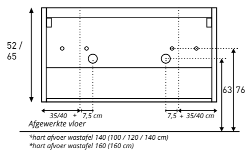
Aan- /afvoer FAKTOR/ASPEKT Dubbel 140 / 160
