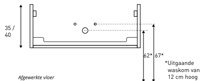
Aan- /afvoer TILO FRAME 60 / 80 / 100
