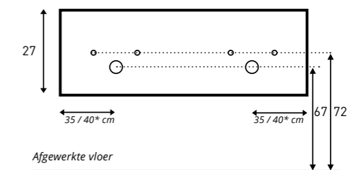
Aan- /afvoer PITCH Dubbel 140 / 160 (designsifon laag model)
