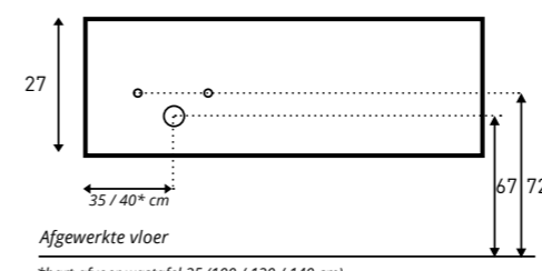
Aan- /afvoer PITCH Links 100 / 120 / 140 / 160 (designsifon laag model)
