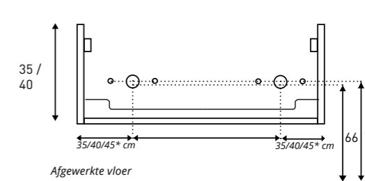
Aan- /afvoer PITCH Dubbel 140 / 160 / 180
