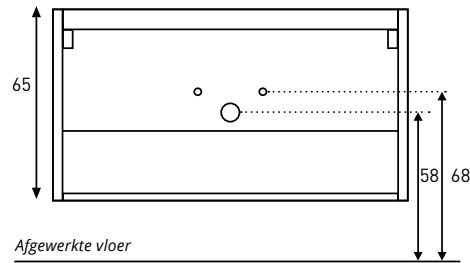
Achteraanzicht tbv aan- /afvoer MOMENTO 80 / 90 / 100 / 120 / 140 / 160 / 180
