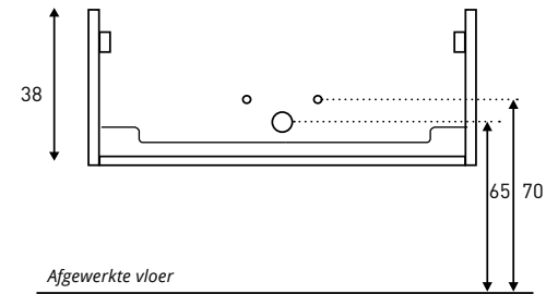
Aan- /afvoer MOMENTO 80 / 90 / 100 / 120 / 140 / 160 / 180
