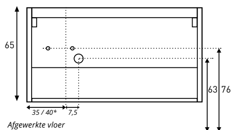
Achteraanzicht tbv aan- /afvoer FAKTOR/ASPEKT LINKS 100 / 120 / 140 / 160
