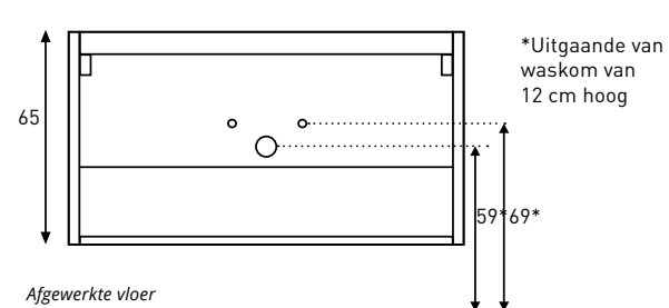
Aan- /afvoer TOPDECK 45 60 / 70 / 80 / 90 / 100 / 120 / 140 / 180
