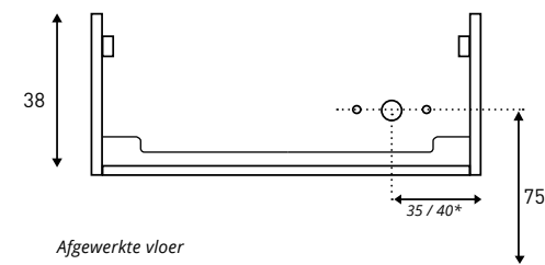
Aan- /afvoer FAKTOR/ASPEKT RECHTS 100 / 120 / 140 / 160 (bijgeleverde platte sifon)
