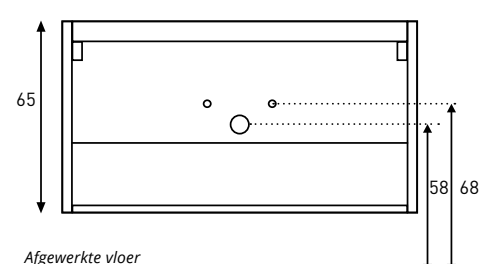
Achteraanzicht tbv aan- /afvoer UNLIMITED 80 / 90 / 100 / 120 / 140
