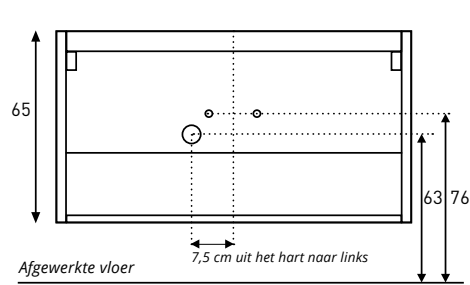
Achteraanzicht tbv aan- /afvoer FAKTOR/ASPEKT MIDDEN 80 / 100 / 120 / 140
