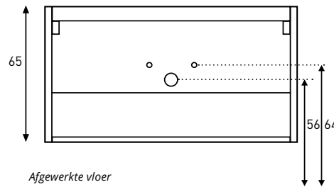
Achteraanzicht tbv aan- /afvoer TABLET 90 / 100 / 120 / 140
