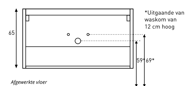
Aan- /afvoer TILO FRAME 100 / 120 / 140 / 160 / 180
