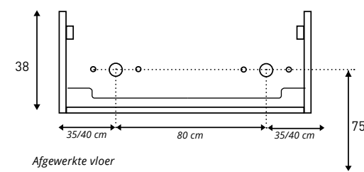
Aan- /afvoer FAKTOR/ASPEKT DOUBBEL 140 / 160 (bijgeleverde platte sifon)
