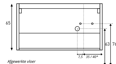
Achteraanzicht tbv aan- /afvoer FAKTOR/ASPEKT RECHTS 100 / 120 / 140 / 160
