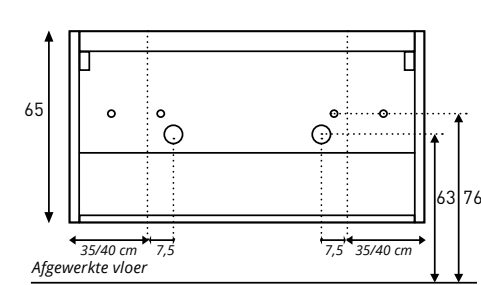
Achteraanzicht tbv aan- /afvoer FAKTOR/ASPEKT DUBBEL 140/160
