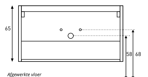
Achteraanzicht tbv aan- /afvoer UNITED 80 / 90 / 100 / 120 / 140
