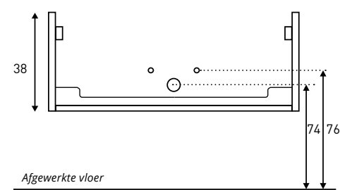
Aan- /afvoer KRAFT 80 / 90 / 100 / 120 / 140 / 160 / 180 (bijgeleverde platte sifon)
