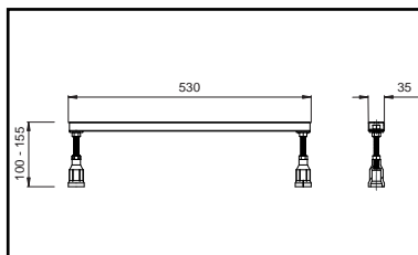
BADPOTEN □ voor inbouwbaden
